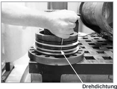
Drehdichtung
