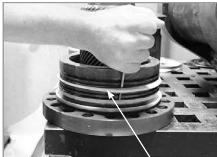
Drehdichtung
