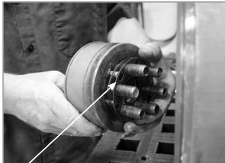
Ausgleichsscheibe
